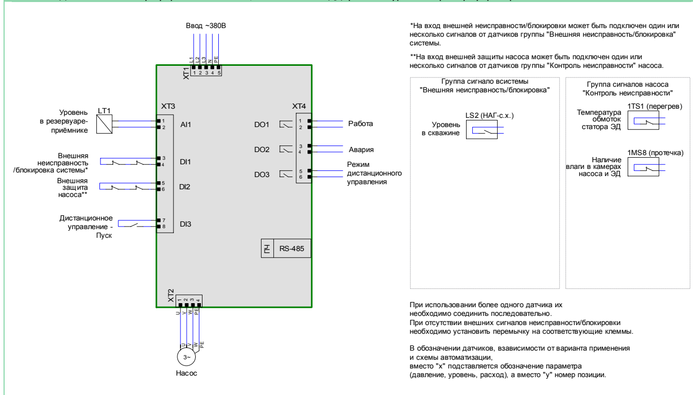
Схема подключений шкафа управления UG03, скважина - поддержание уровня в резервуаре-приёмнике
