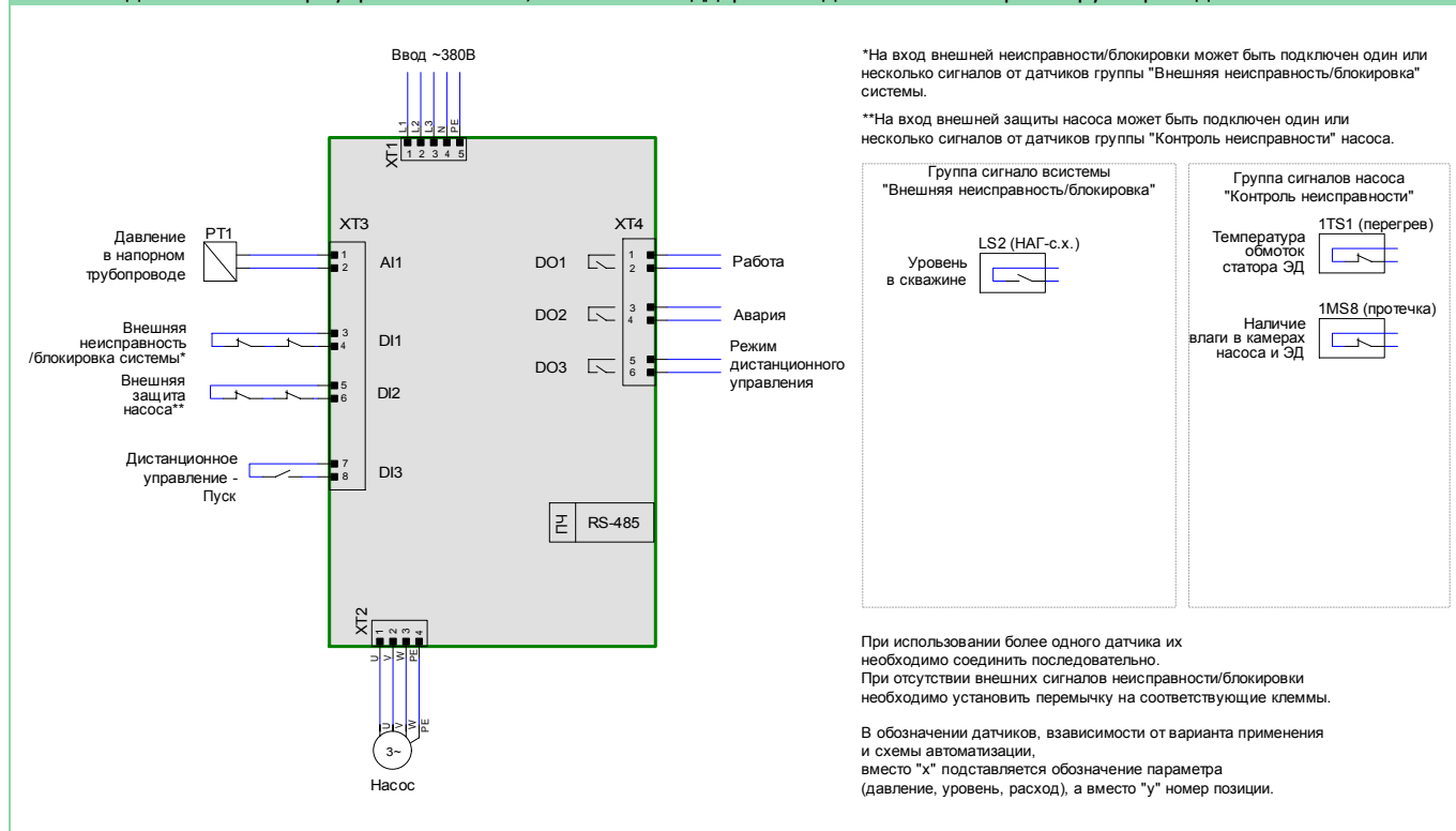
Схема подключений шкафа управления UG03, скважина - поддержание давления в напорном трубопроводе
