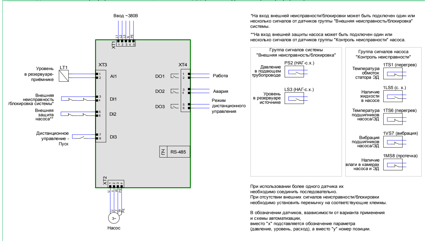
Схема подключений шкафа управления UG03, система поддержания уровня в резервуаре-приёмнике
