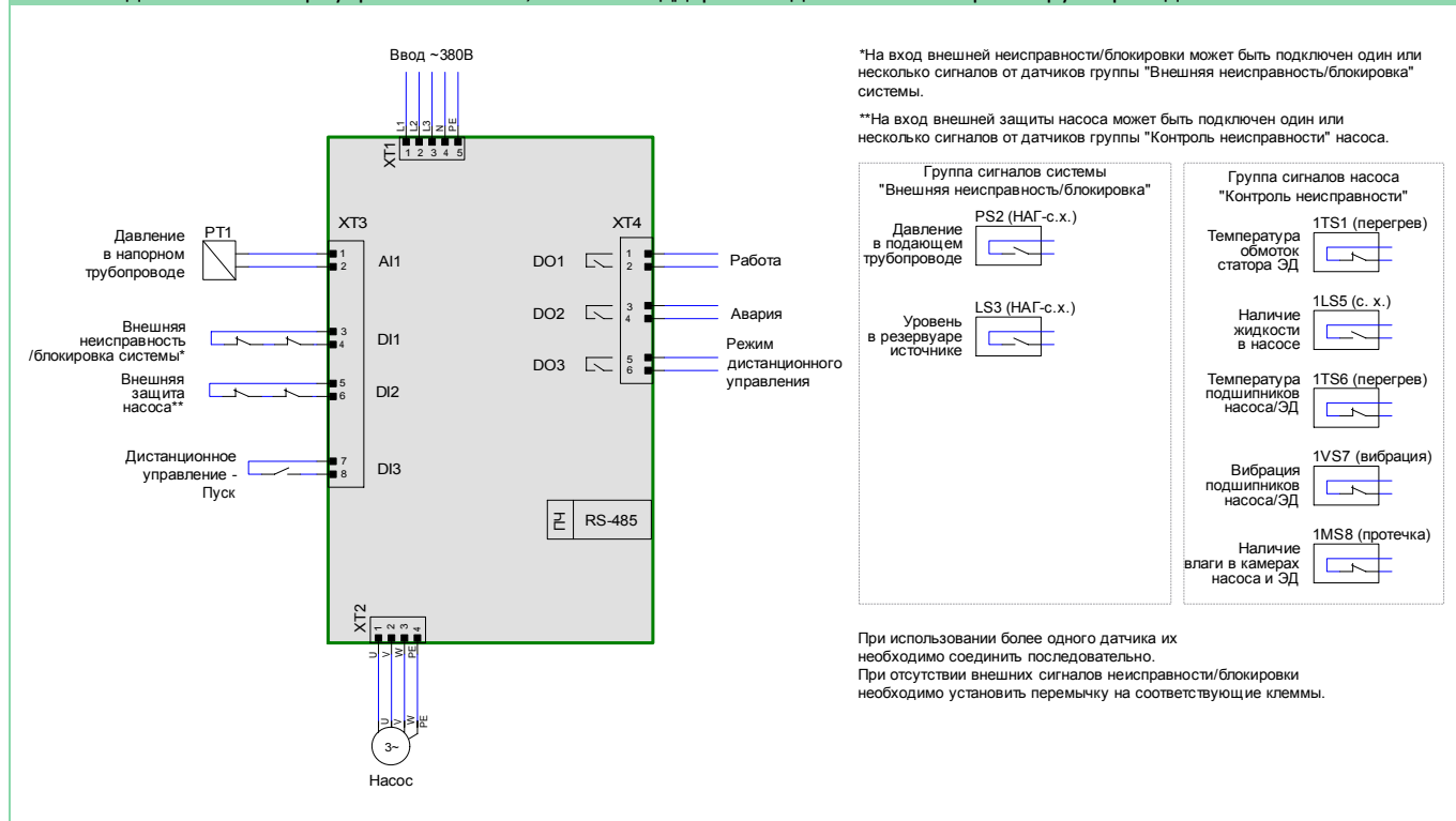
Схема подключений шкафа управления UG03, система поддержания давления в напорном трубопроводе
