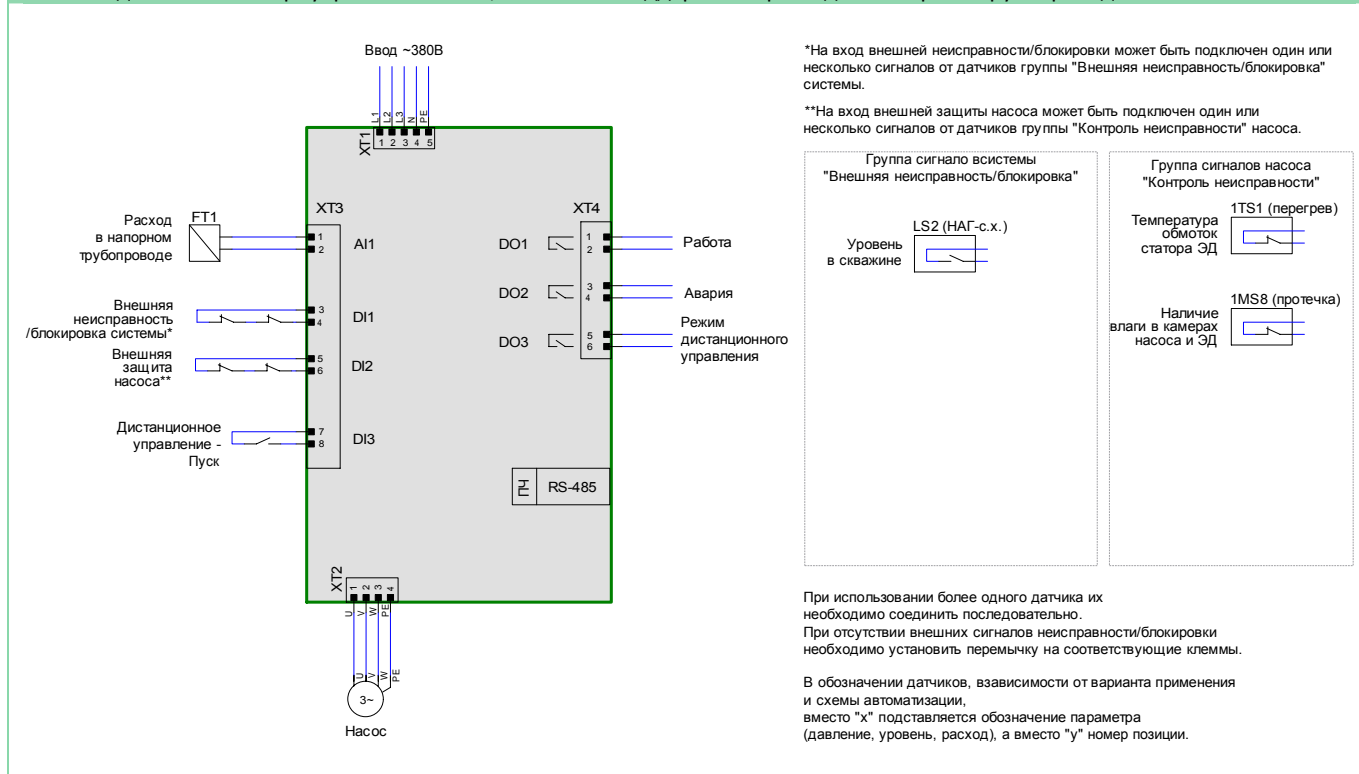
Схема подключений шкафа управления UG03, скважина - поддержание расхода в напорном трубопроводе
