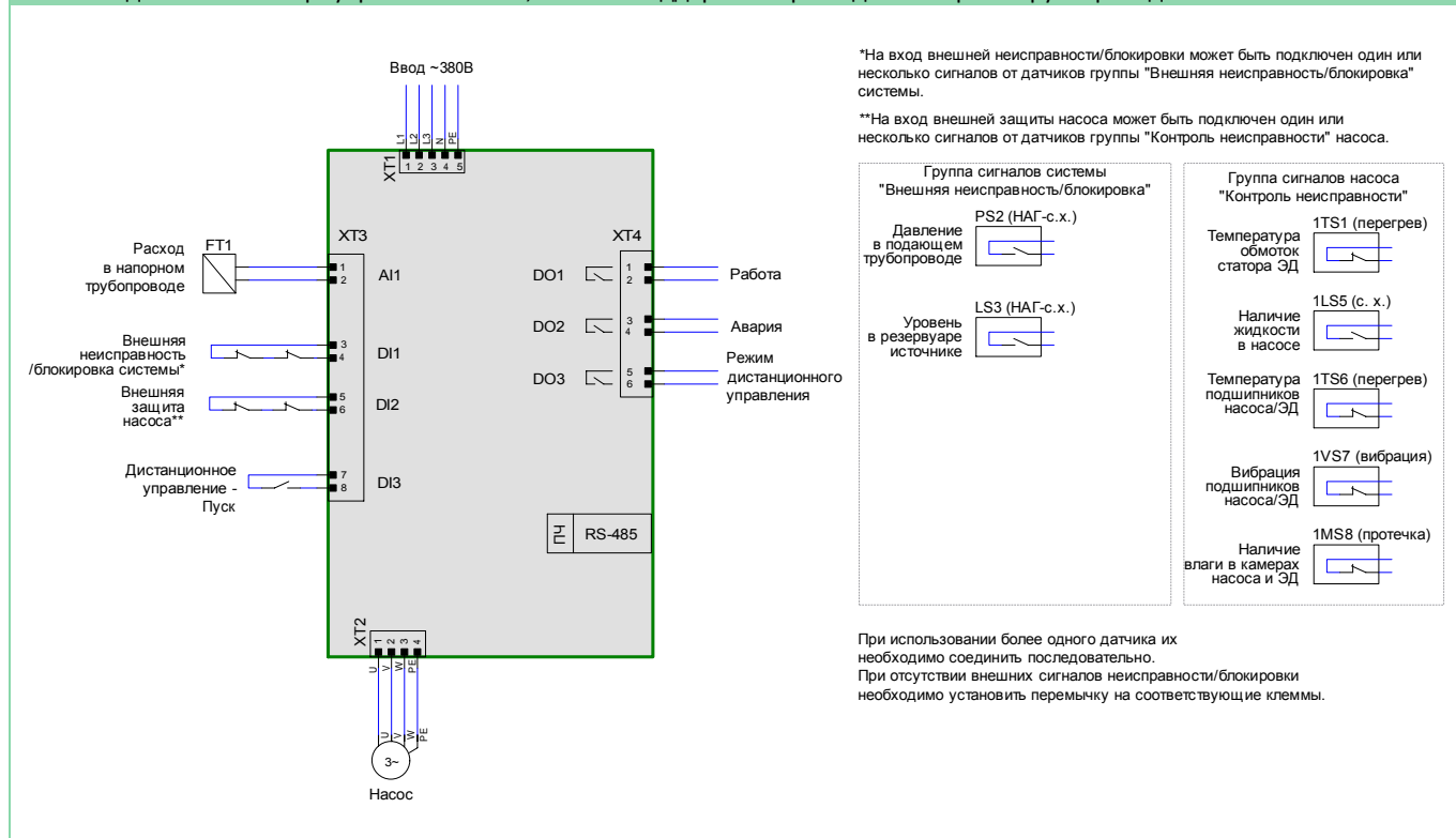
Схема подключений шкафа управления UG03, система поддержания расхода в напорном трубопроводе
