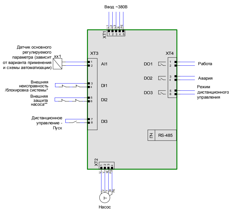
Общая таблица подключений шкафов управления UG03 (1)
