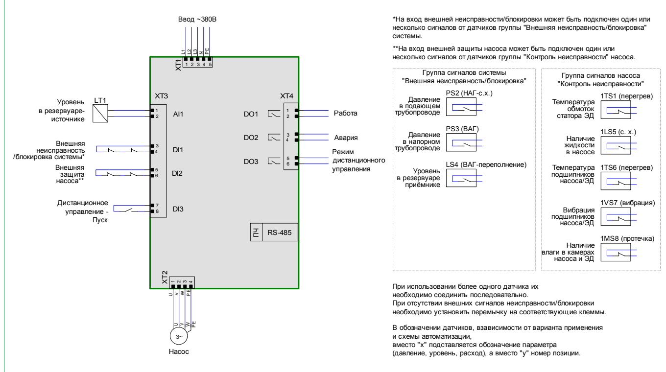
Схема подключений шкафа управления UG03, система поддержания уровня в резервуаре-источнике
