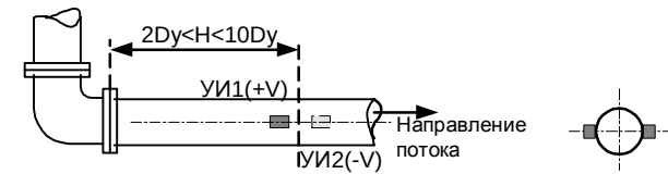
Установка ПП-1 после "колена"
