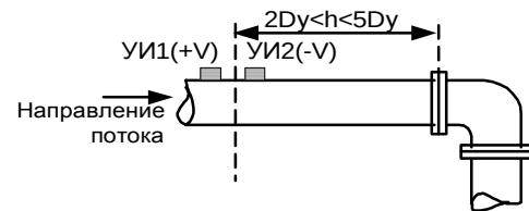
Установка ПП-1 до "колена"
