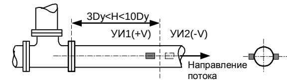
Установка ПП-1 после "тройника"
